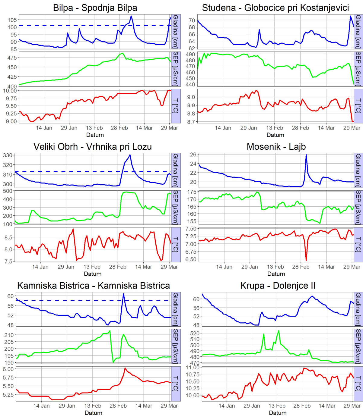
Slika 3. Nihanje vodne gladine (modro), temperature (rdeče) in specifične električne prevodnosti (zeleno) na izbranih merilnih mestih kraških izvirov med januarjem in marcem 2020
