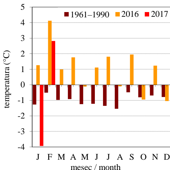
Slika 7. Odklon mesečne povprečne temperature zraka od povprečja primerjalnega obdobja 1981–2010 Figure 7. Deviation of monthly mean air temperature from reference period 1981–2010
